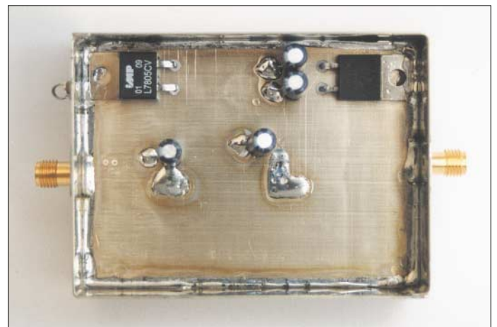
Bild 1: Alle SMD-Bauelemente verlötet man auf der Leiterseite der Platine.
