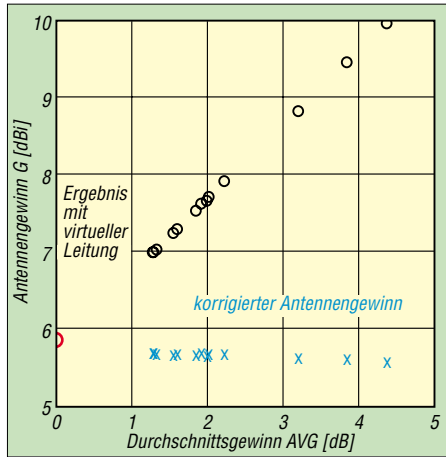
Bild: 7 Antennengewinn G in dBi und korrigierter Antennengewinn G_{\text{korr}} = G - AVG , aufgetragen über dem Durchschnittsgewinn AVG. Die Zahlenwerte stammen aus einer Dipolsimulation mit angeschlossener Zweidrahtleitung, siehe Tabelle 1.
