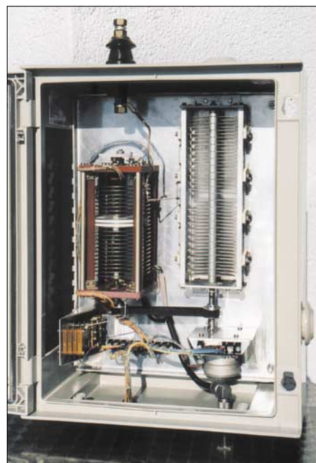
Bild 3: Antennentuner im spritzwassergeschützten Gehäuse, rechts unten Motor und Getriebe, oben der Antennenanschluss
