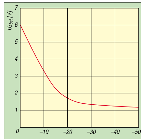
Bild 3: Dämpfungen größer als 20 dB sind erst bei Abstimmspannungen unter 1,76 V erreichbar, sodass der Hauptnutzungsbereich zwischen 1 und 2 V liegt. Dies erfordert eine möglichst genau einstellbare Spannungsquelle mit Anzeigeinstrument oder die Ansteuerung per Software.
