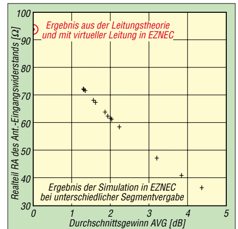
Bild 6: Realteil RA des Antenneneingangswiderstands in \Omega , aufgetragen über dem Durchschnittsgewinn AVG. Die Zahlenwerte stammen aus einer Dipolsimulation mit angeschlossener Zweidrahtleitung, siehe Tabelle 1. Eine verbindende Kurve lässt sich ohne Probleme auf den Wert bei \text{AVG} = 0 \text{ dB} extrapolieren und erreicht dort den wahren Wert RA = 94 \Omega .
