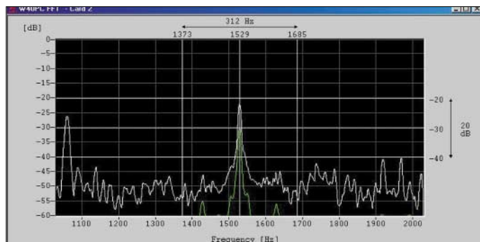
Bild 5: So sollte der Träger eines fabrikneuen Gerätes aussehen, wenn sich die Ionosphäre im Normalzustand befindet. Screenshots: DK20M
