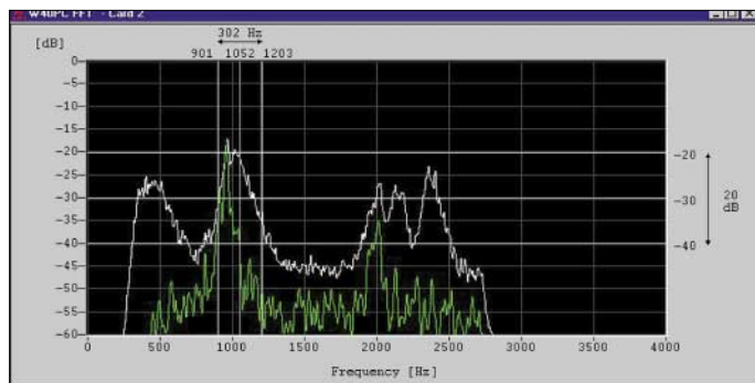
Bild 1: Sonagramm eines via Aurora reflektierten CW-Signals
