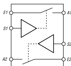
Bild 1: MAX4541 als Blockschaltbild
